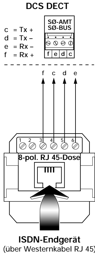
Skizze: „S 0 -AMT/S 0 -BUS“ als interner Mehrgeräteanschluß
