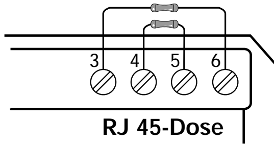
Skizze: Anklemmen der 100 Ohm-Abschlußwiderstände
