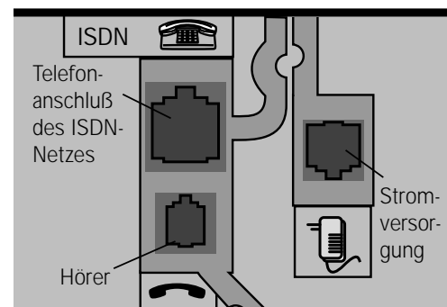
Unterseite des Gerätes
