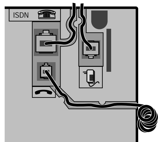
Unterseite des Gerätes
